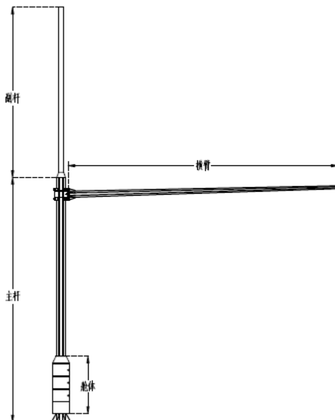
图2 智慧多功能杆杆体组成示意图
